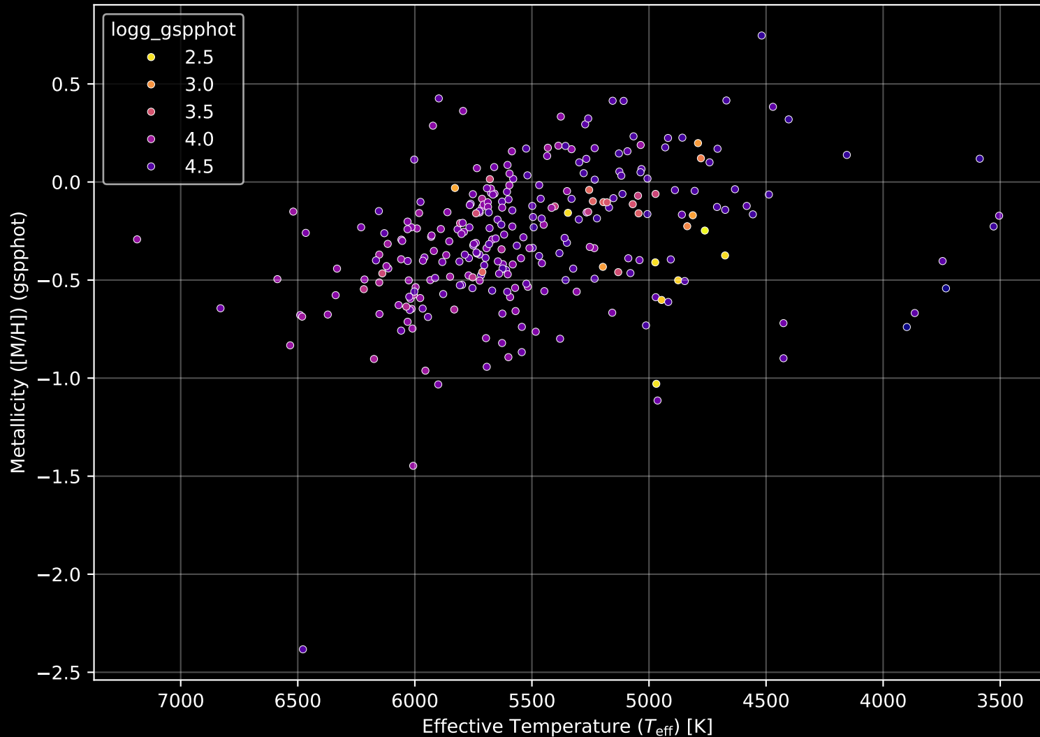
GALAH DR4 Field: [6922] Stellar Population Parameters (n= 284)
