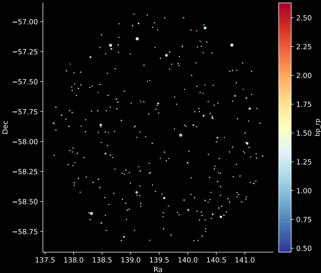
GALAH DR4 Field: [6922] Stars: 284
