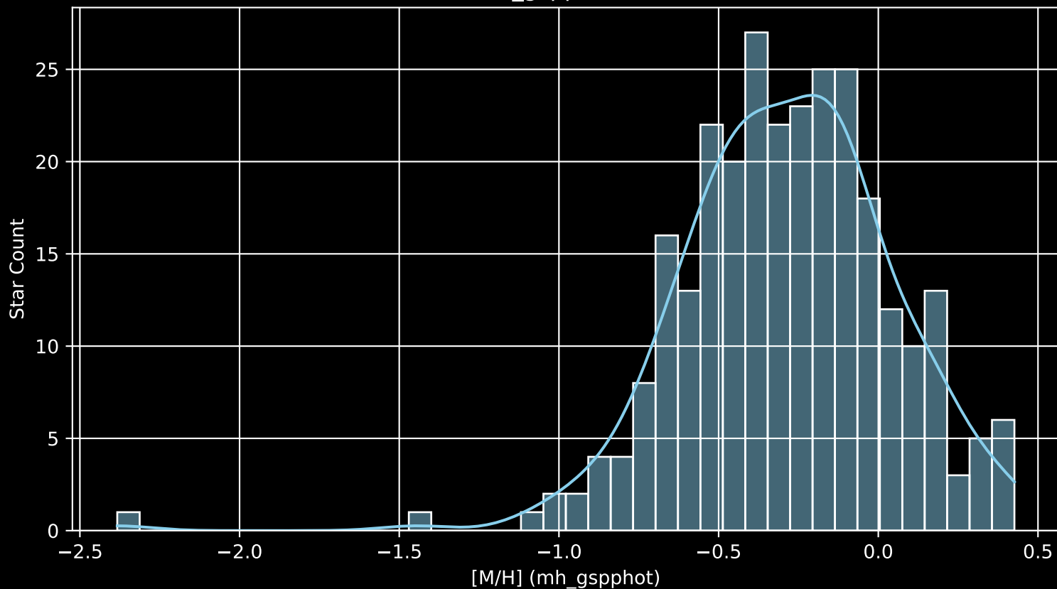
GALAH DR4 Field: [6922] [M/H] (mh_gspphot) (n= 283)
